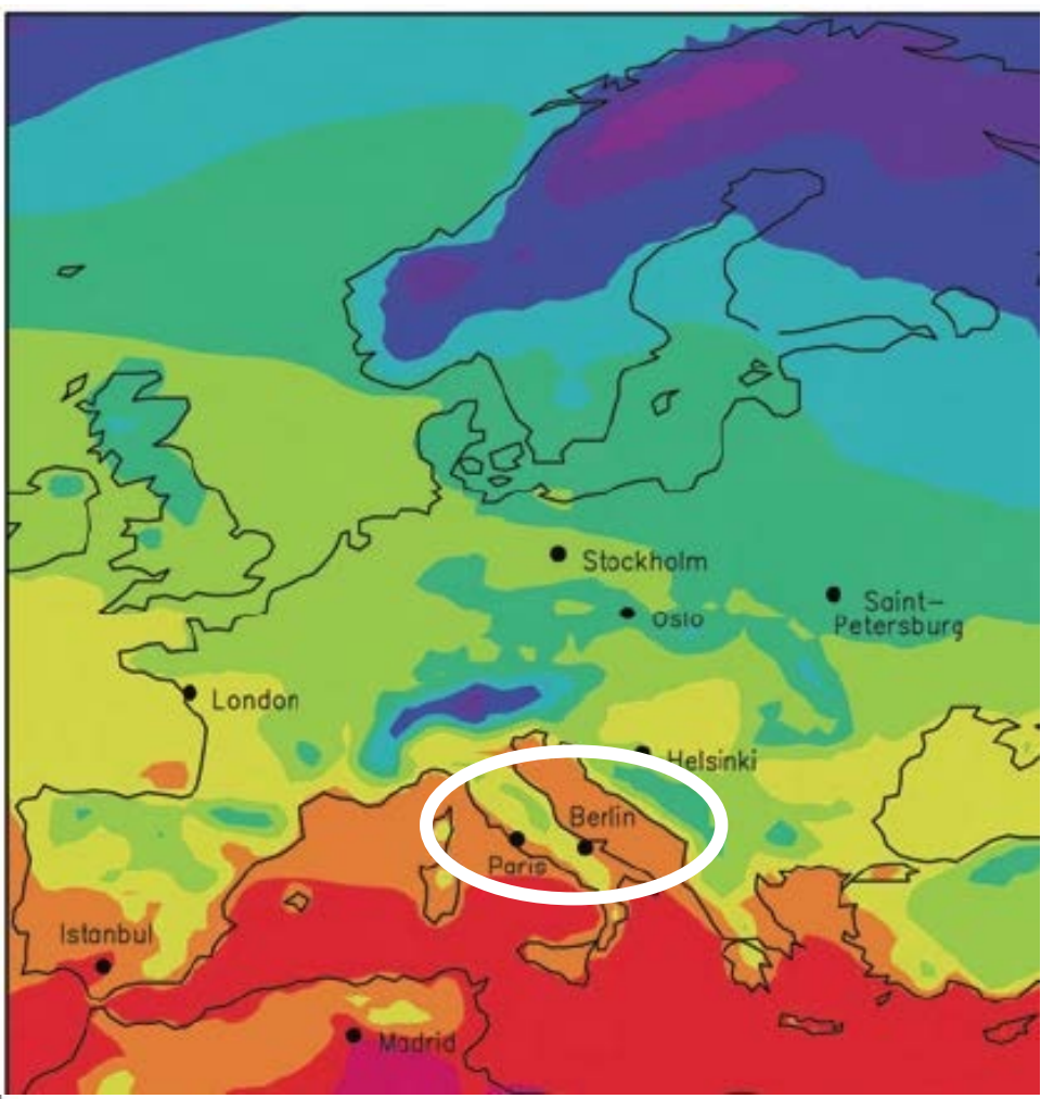
Météo-France Center model, ARPEGE-Climat , Emission scenario SRES/A2
